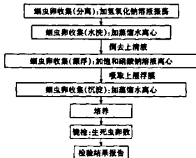
图 D1 污泥中蛔虫卵检验程序
